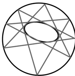
FIGURE 20.8. Poncelet’s Porism 20.10.8
