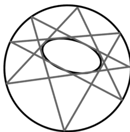
FIGURE 19.8. Poncelet’s Porism 19.10.8
